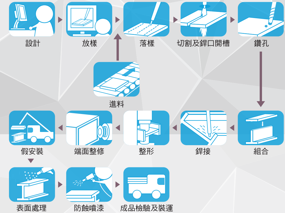
中鋼構製程流程圖
